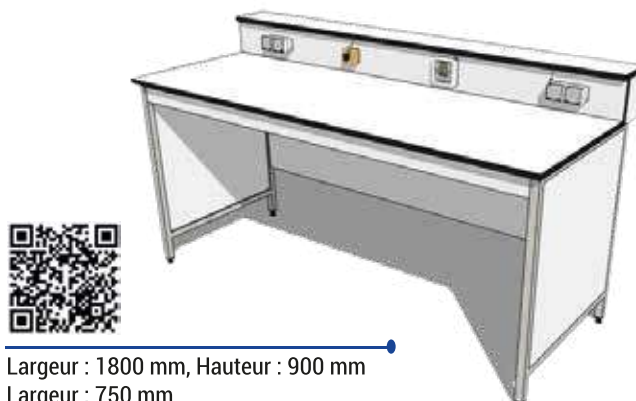
PL04 PAILLASSE DE LABORATOIRE SÈCHE AVEC ALIMENTATION ÉLECTRIQUE
